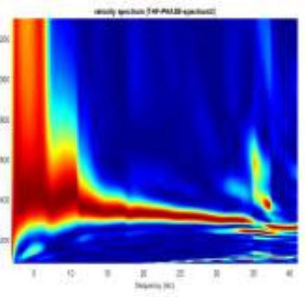
MASW spettro THF
