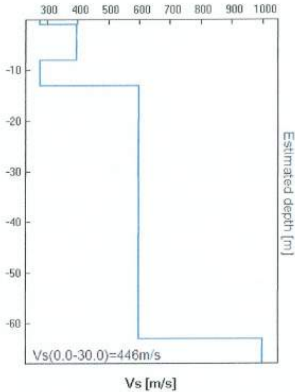
Profilo di velocità delle onde di taglio ( V_s ) ottenuto
